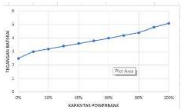
Gambar 4. Grafik Kapasitas SOC (State of Charge) Baterai
